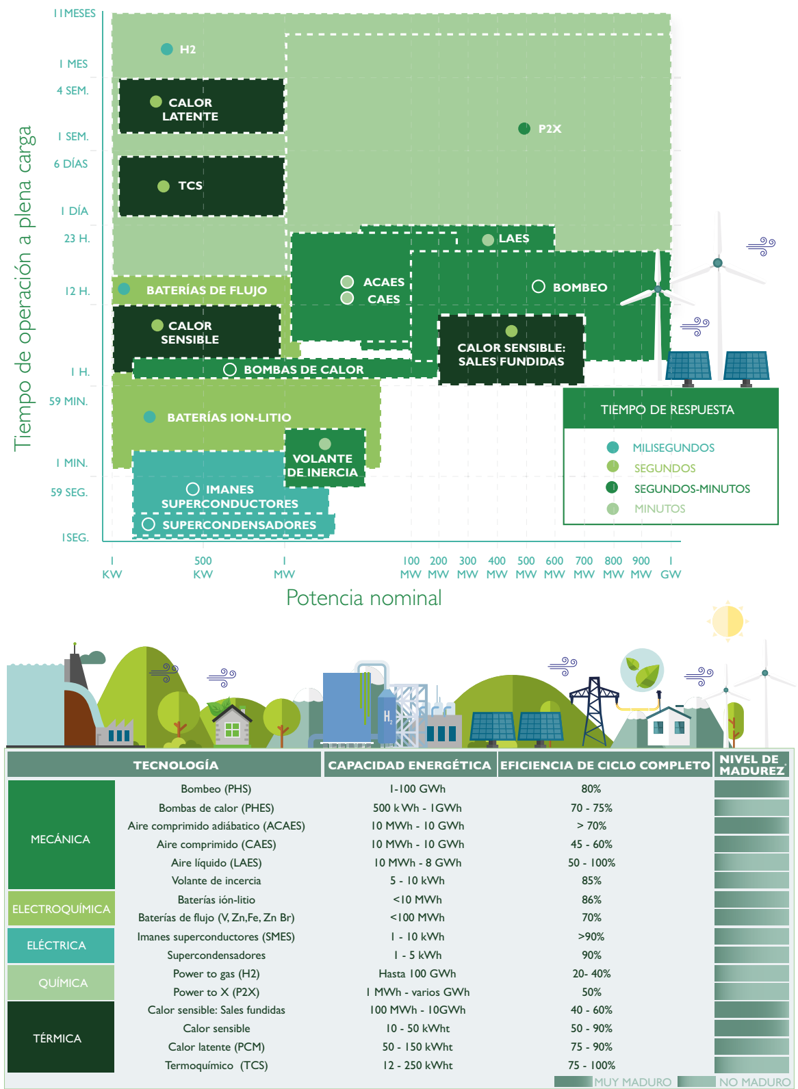
FIGURA 3. Parámetros de funcionamiento de las tecnologías de almacenamiento energético
